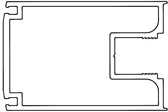
CI-5027 Pivot Stile
