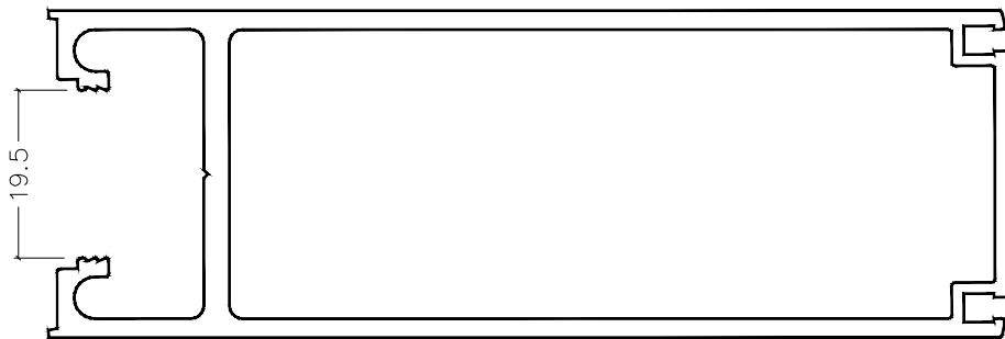
CI-6037 Wide Pivot Stile
