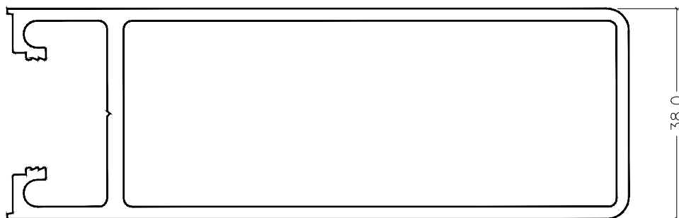
CI-6038 Wide Plain Stile
