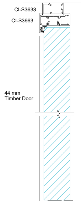
SVELTE 36 Aluminium Hinged Door (Barwon)
