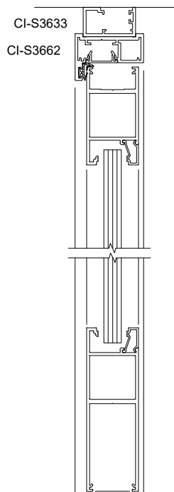
SVELTE 36 Aluminium Hinged Door (Barwon)
