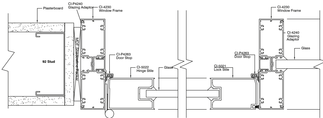
Platinum 120 Aluminium Hinge Door
