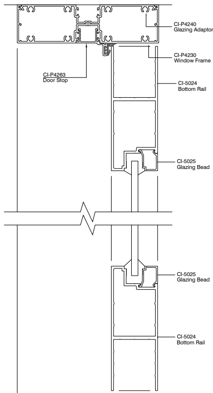
Platinum 120 Aluminium Hinge Door
