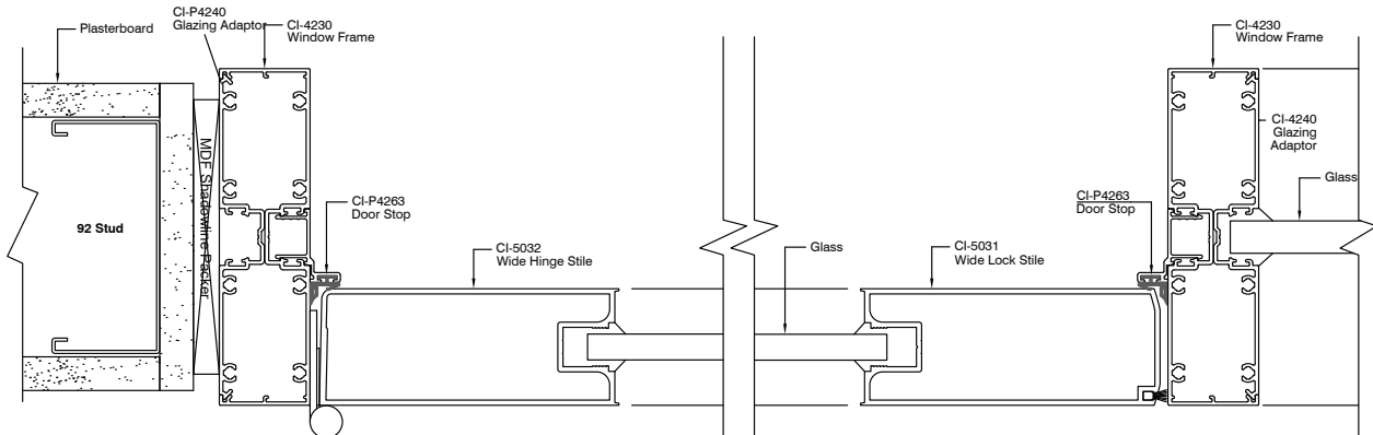
Platinum 120 Aluminium Wide Hinge Door
