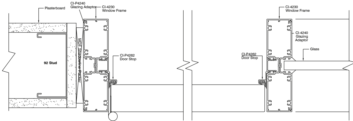
Platinum 120 Timber Hinge Door
