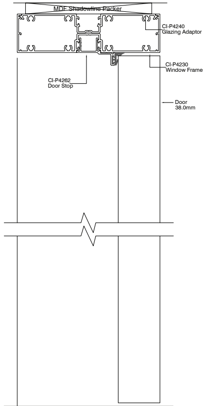
Platinum 120 Timber Hinge Door
