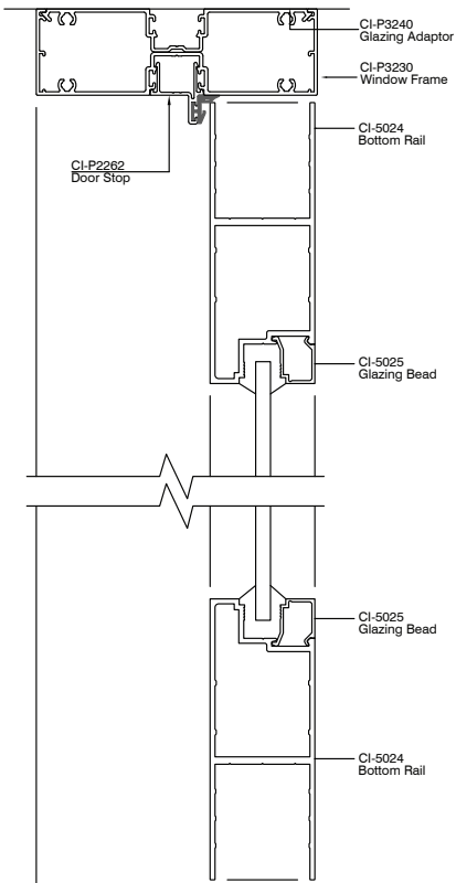
Platinum 105 Aluminium Hinge Door
