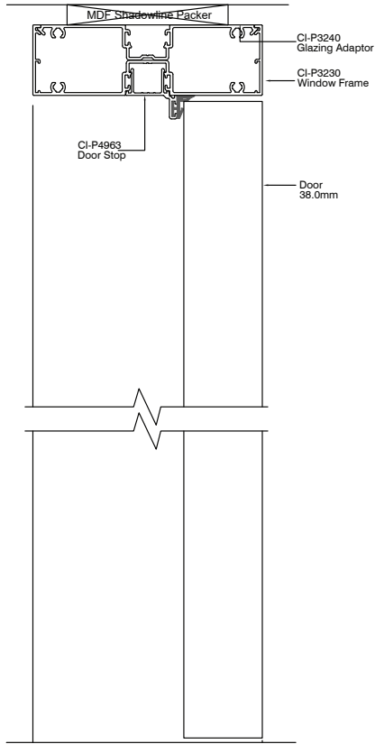
Platinum 105 Timber Hinge Door
