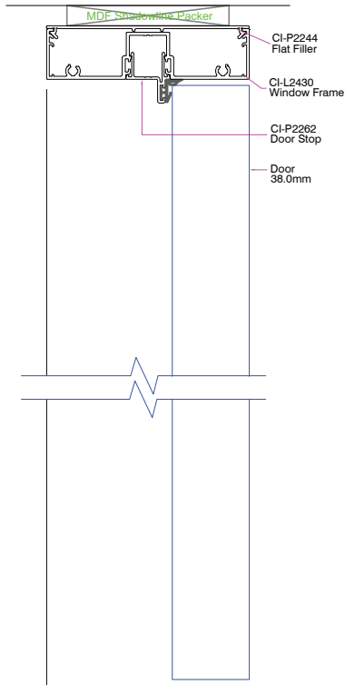
Linium 90 Aluminium Hinge Door
