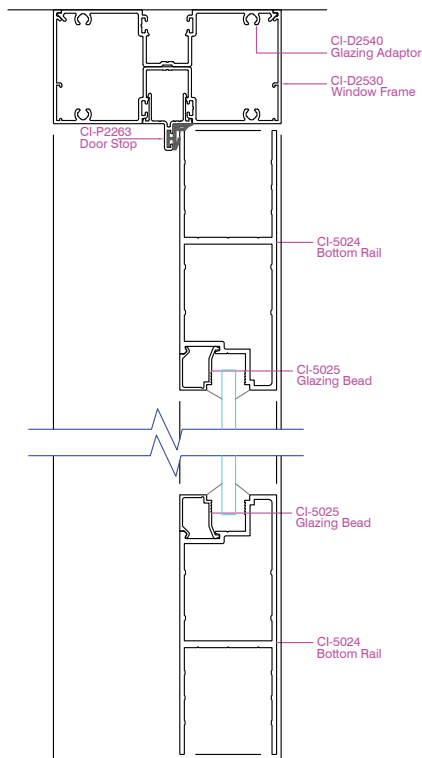
Definium 90 Aluminium Hinge Door
