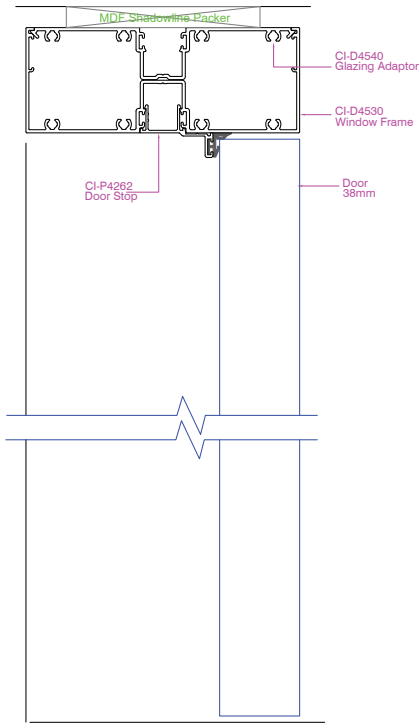
Definium 120 Aluminium Hinge Door
