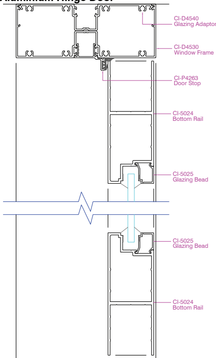
Definium 120 Aluminium Hinge Door
