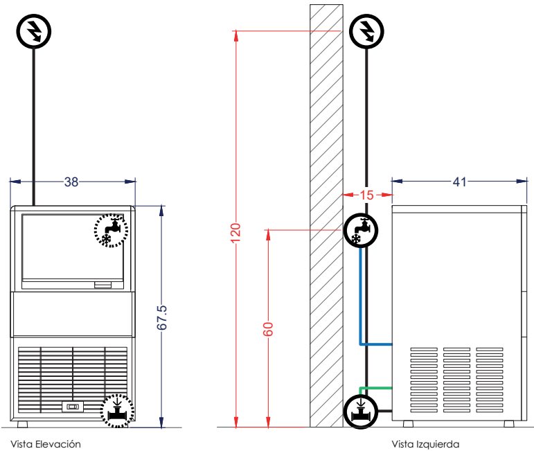
Vista Elevación
