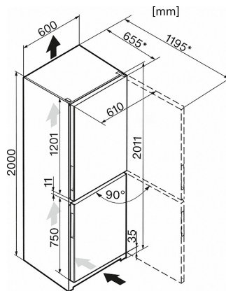
KFN 29132 D ws + edt/cs, KFN 29133 D ws + edt/cs, KFN 29162 D ws + edt/cs Serie 120 (croquis) (*nota al pie de página)
