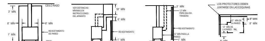
PARED SENCILLA PROTEGIDA
