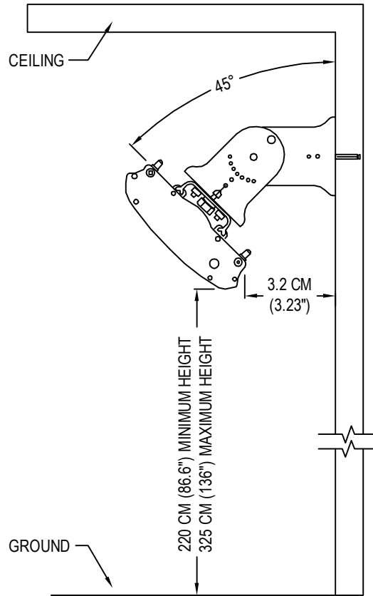
END ELEVATION
