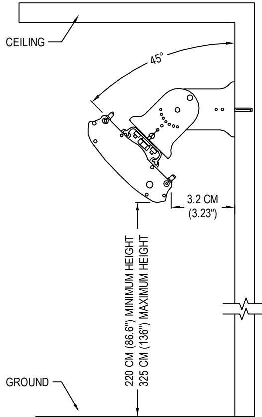
END ELEVATION
