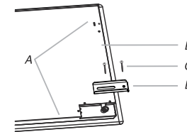
A. 前面或后面安装连接螺钉孔的位置 B. 灶具底盘底部 C. 连接螺钉 D. 安装支架(建议终端位置)
