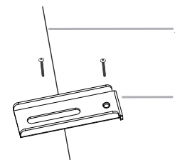
A. Partie inférieure de la base du bord de la table de cuisson B. Bride de fixation
