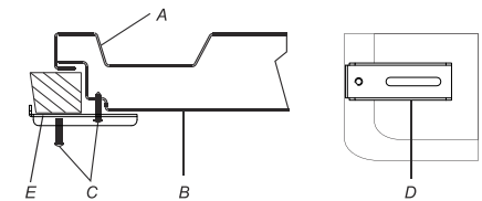
A. 灶具 B. 灶具底盘 C. 2英寸(5.1厘米)连接支架螺 D. 安装支架(延伸到超过灶具底部最远可 允许安装连接螺钉的位置) E. 灶台
