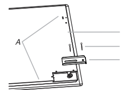
A. Trous de vis d'attache pour emplacement facultatif à l'avant et à l'arrière B. Fond de la base de la table de cuisson C. Vis d'attache D. Bride de fixation (emplacements aux extrémités recommandés)
