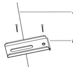
A. 灶具底部的边缘 B. 安装支架
