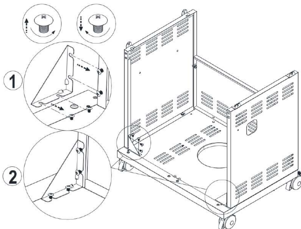
Desatornille hasta la mitad los tornillos en las placas inferior y lateral, luego coloque el soporte triangular en los orificios de los tornillos correspondientes y atornille firmemente. Figura 4
