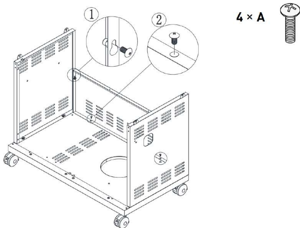
Instale el panel trasero, la parte inferior en el lugar correspondiente con cuatro tornillos A. Figura 3
