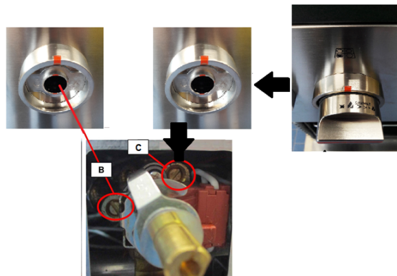
Figure 3: Le robinet du brûleur à double flamme
