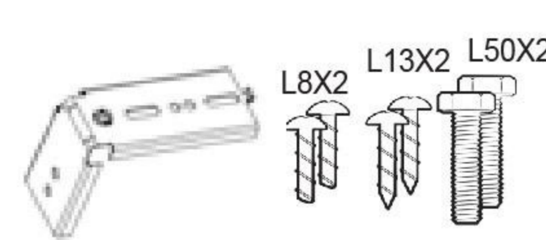
Soporte de montaje en panel (2) Tomillo (6)
