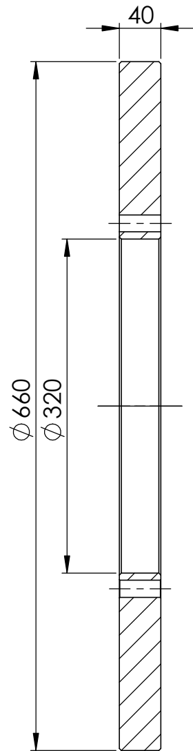
SECTION A-A SCALE 1 : 5
