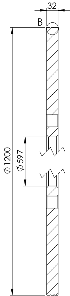
SECTION A-A SCALE 1 : 6
