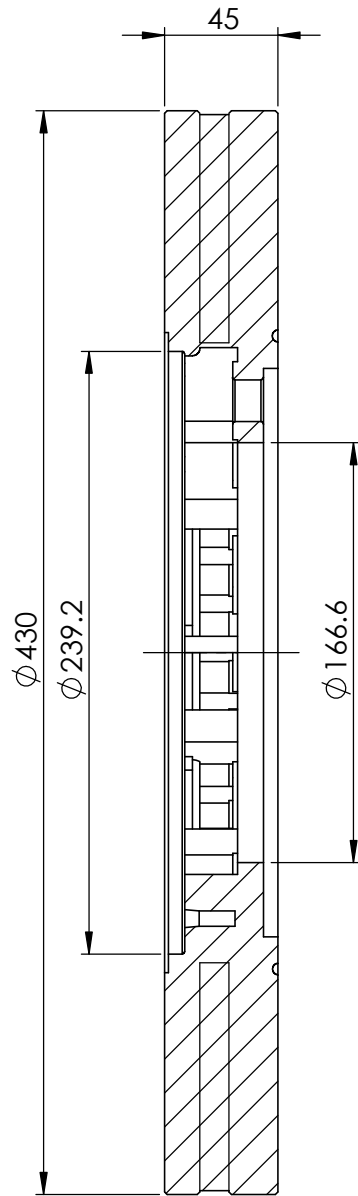
SECTION A-A SCALE 1 : 3
