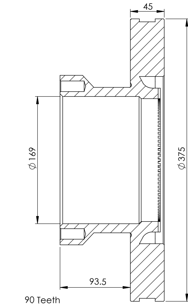
SECTION A-A SCALE 1 : 3
