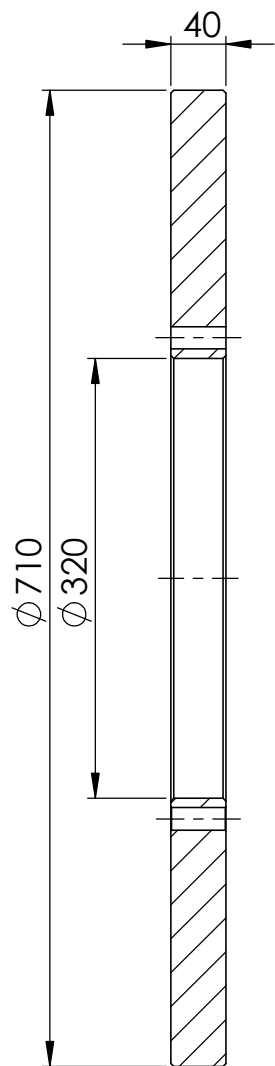
SECTION A-A SCALE 1 : 5.5
