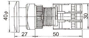
GLBF22-10/C
