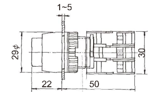
GEBL22-10/C
