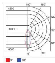
12W-15D-4000K-CRI80
