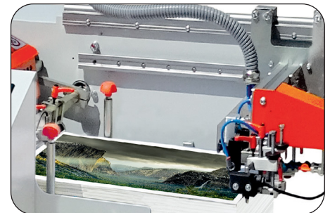
Feeding module
