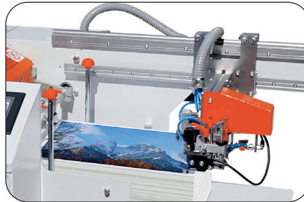
Feeding module
