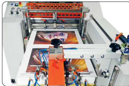
Feeding module
