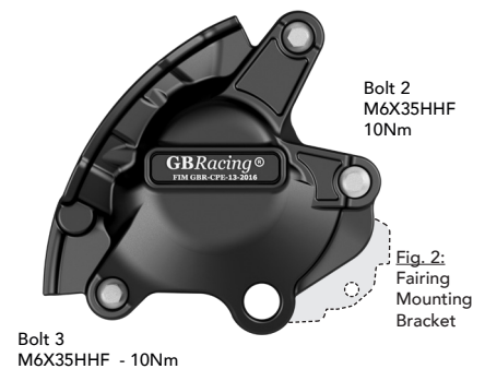
Bolt 1 M6X35HHF - 10Nm - See Fig. 1
