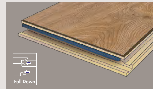
Met het "Fall Down" systeem aan de kopse kant. Avec le système "Fall Down" sur les côtés courts. "Fall Down" system on the butt ends.
