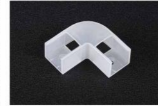
PC接头:613转角 内空尺寸: 17.2*14.4MM
