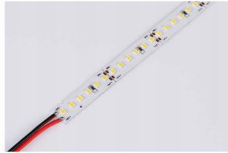
欧司朗灯珠硬灯条 电压: 直流DC12V / 24V(可选) 功率: 16W/米 灯珠: 2835 144珠/米 宽度: 12mm 长度: 1000mm 色温: 3000K/4000K/6000K 显指: RA90
