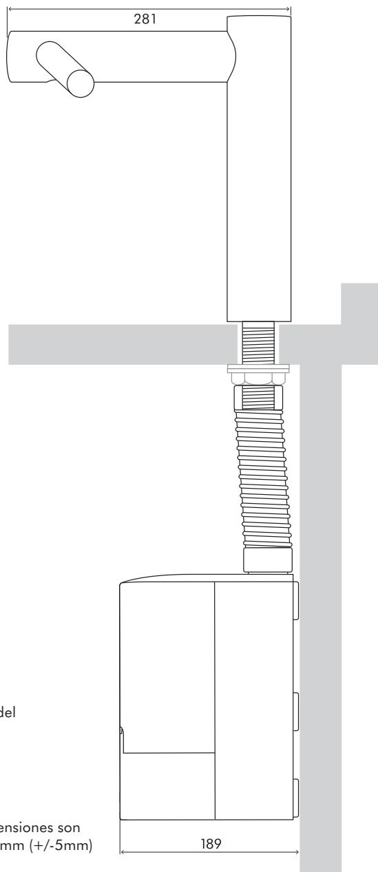
ALZADO LATERAL
