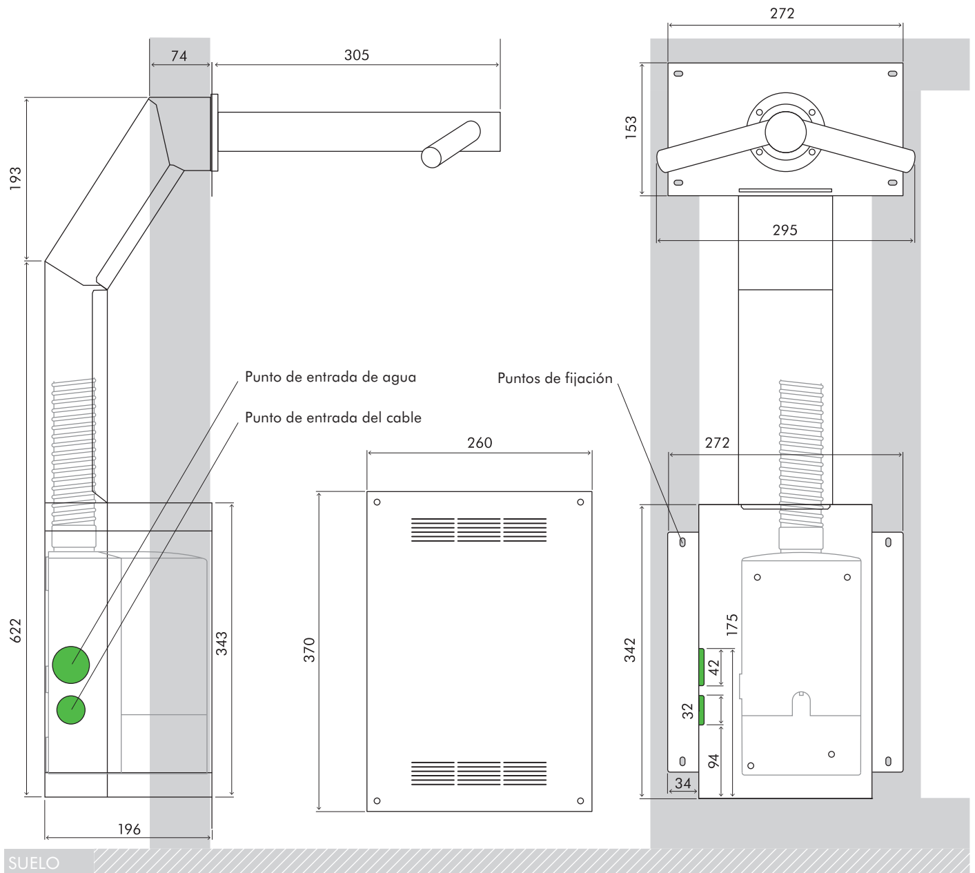
ALZADO LATERAL
