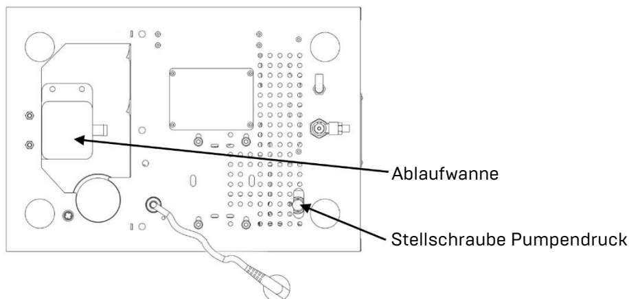
Abb. 5 Unterseite Maschine
