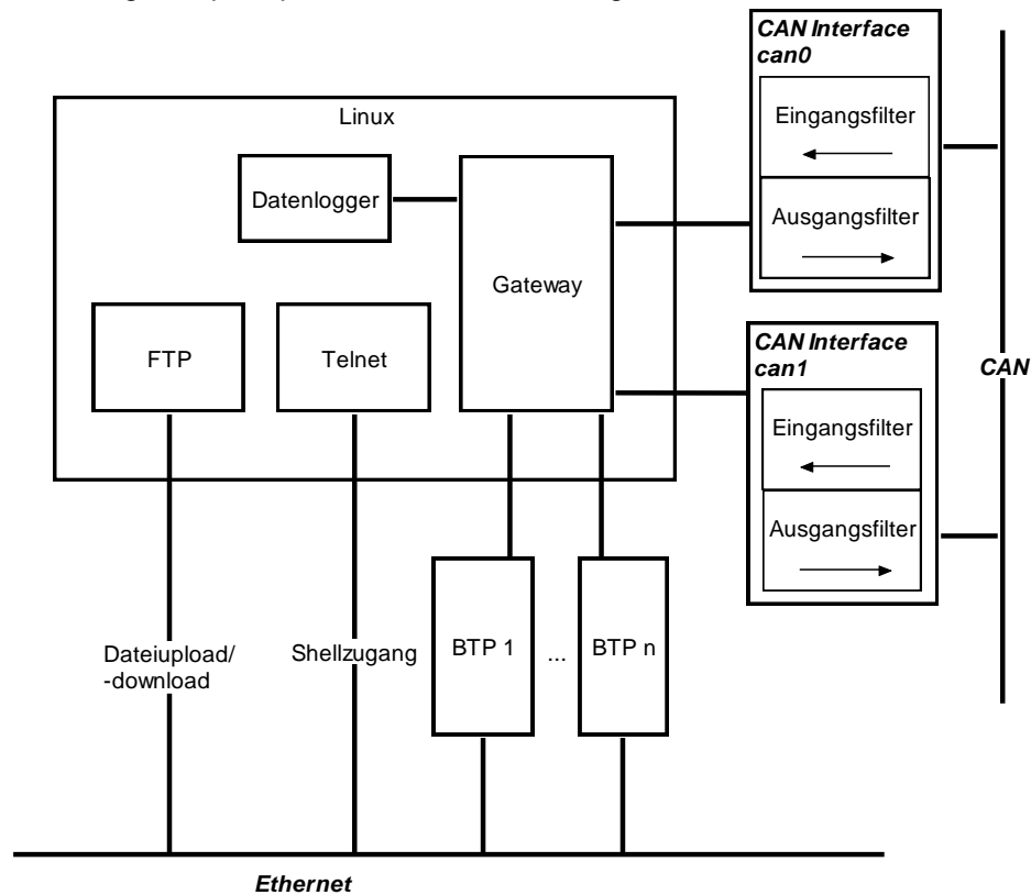
Abbildung 8: Prinzip CAN-Ethernet-Gateway V2
