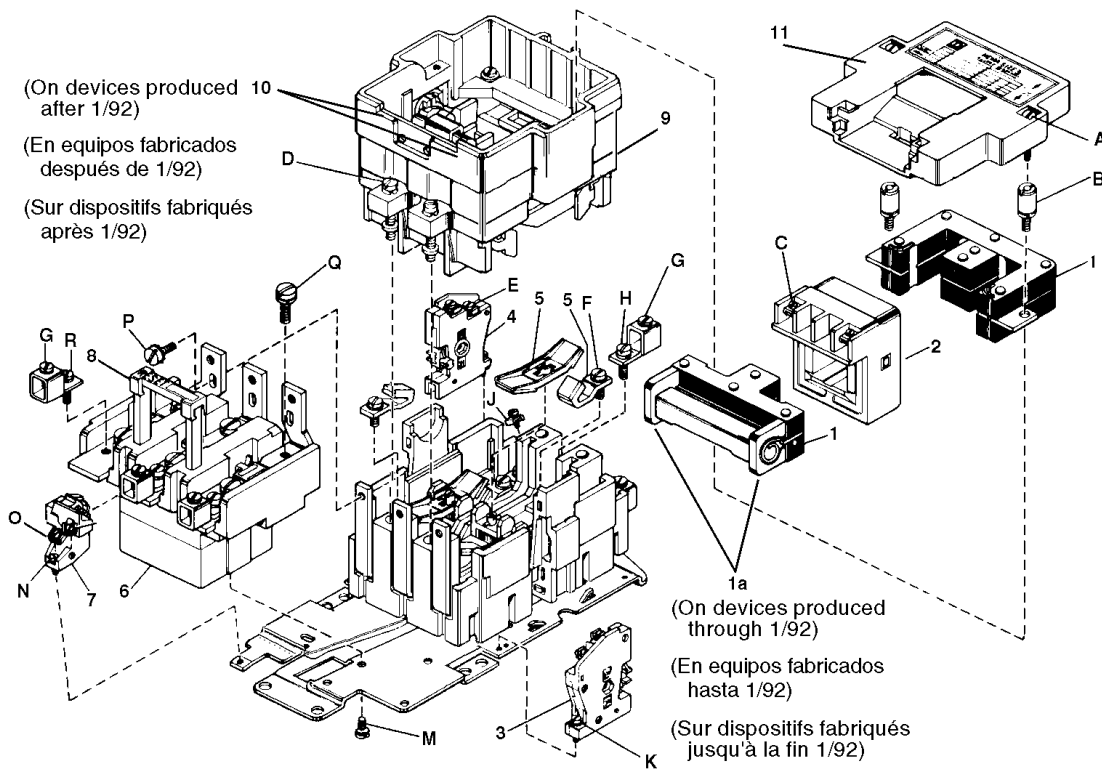
Figure / Figura / Figure 1 : Contactor and Starter Assembly / Ensamble de contactor y arrancador Assemblage de contacteur et de démarreur
