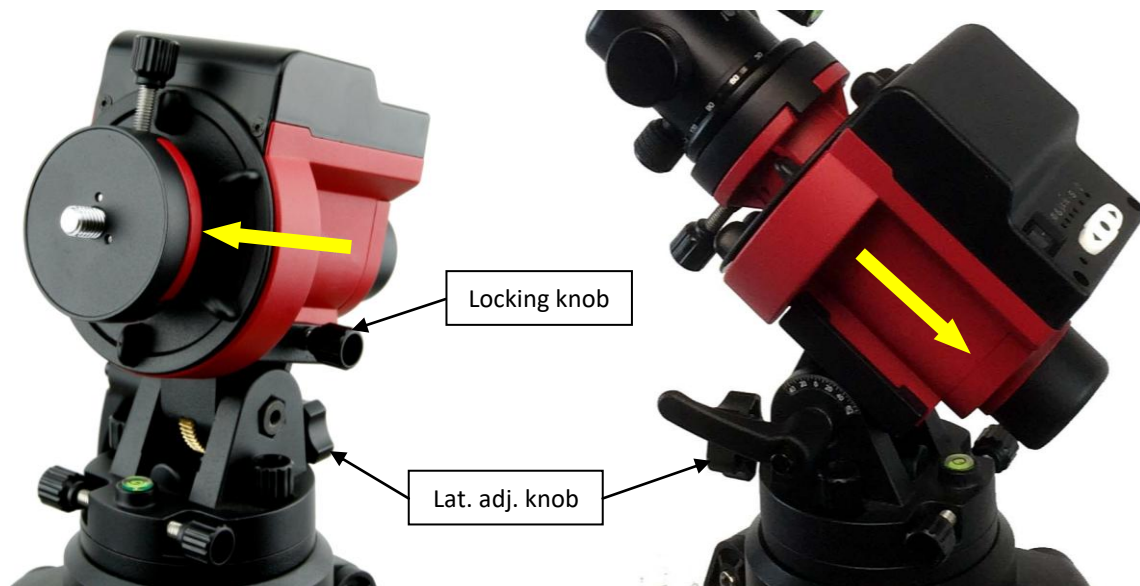
Figure 17. Switch mount head from low latitude to high latitude
