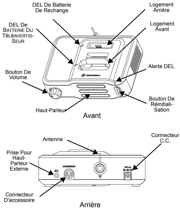
Figure 2 : Chargeur amplificateur
