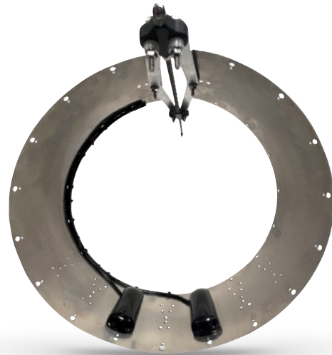
Dual AV Sensor Installation Dual AV Sensors with Band and Screw-Jack
