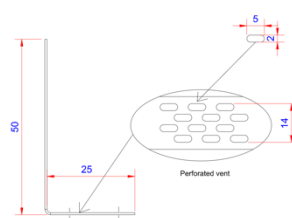
2 VENTILATIONSPROFIL – L TYPE
