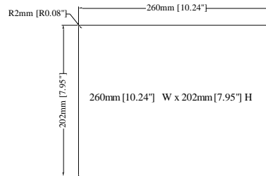
Cutout Dimensions
