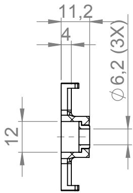
SCHNITT A-A
