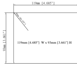
Cutout Dimensions
