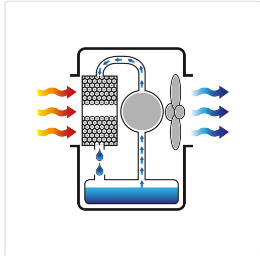
Diagramma di raffreddamento evaporativo Master
