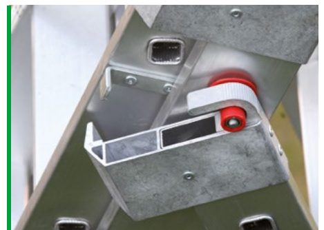
Possibilità di utilizzo come scala zoppa. Can be adjusted to use on stairs.
