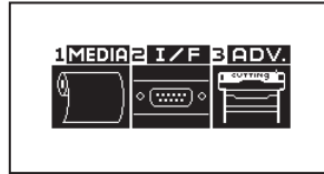
Simple mode
