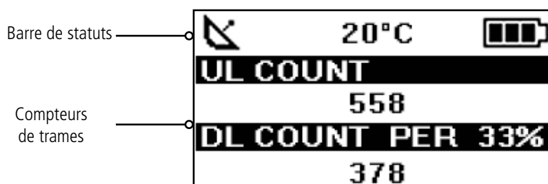
Figure 11 : Ecran PER
