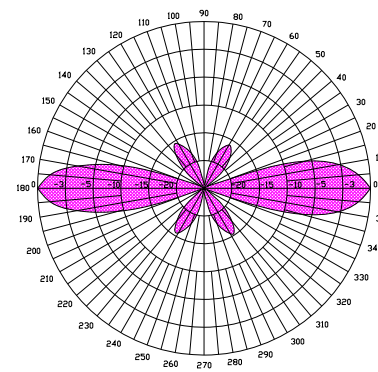
垂直方向图
