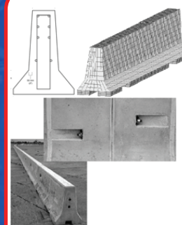
Road/Jersey Barriers Load & Pin • JJ Hook • Bolt Specify type
