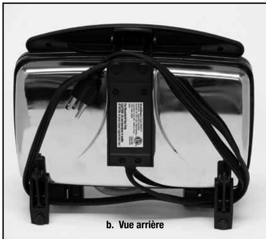
Figure 3. Le câble s'insère facilement sous le WafflePro® classique pour un rangement vertical comme illustré.
