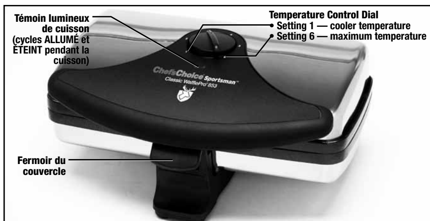
Figure 1. WafflePro® classique.
