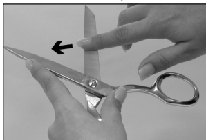
Рисунок 12: Осторожно найдите заусенец на протяжении всей длины задней поверхности лезвия. Обратите внимание на стрелку, указывающую направление движения пальца при касании лезвия.
