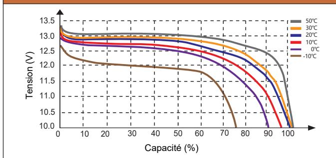
COURBE DE DÉCHARGE À TEMPÉRATURE DIFFÉRENTE (0.5C)
