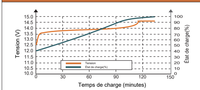
COURBE D'ÉTAT DE CHARGE (0.5C, 25°C)
