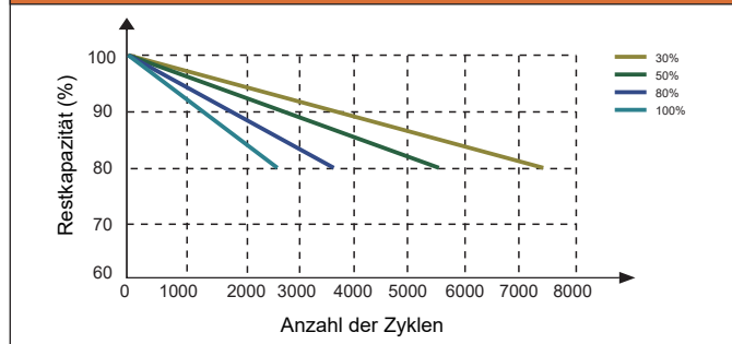
UNTERSCHIEDLICHE DOD-ENTLADUNGSZYKLUS-LEBENS-KURVE
