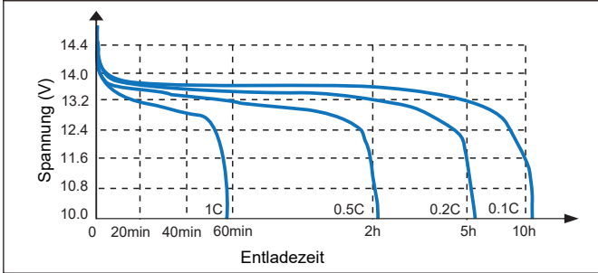
ENTLADEKURVE MIT UNTERSCHIEDLICHER RATE (25°C)
